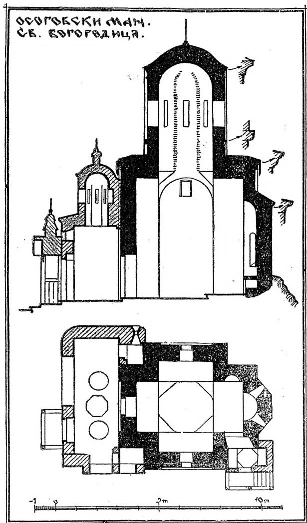
Сл 10 — Основа и уздужни пресек старе цркве у манастиру Осогову.
