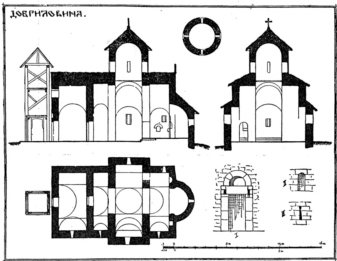
Сл. 1. — Основа и пресеци цркве манастира Добриловине.
