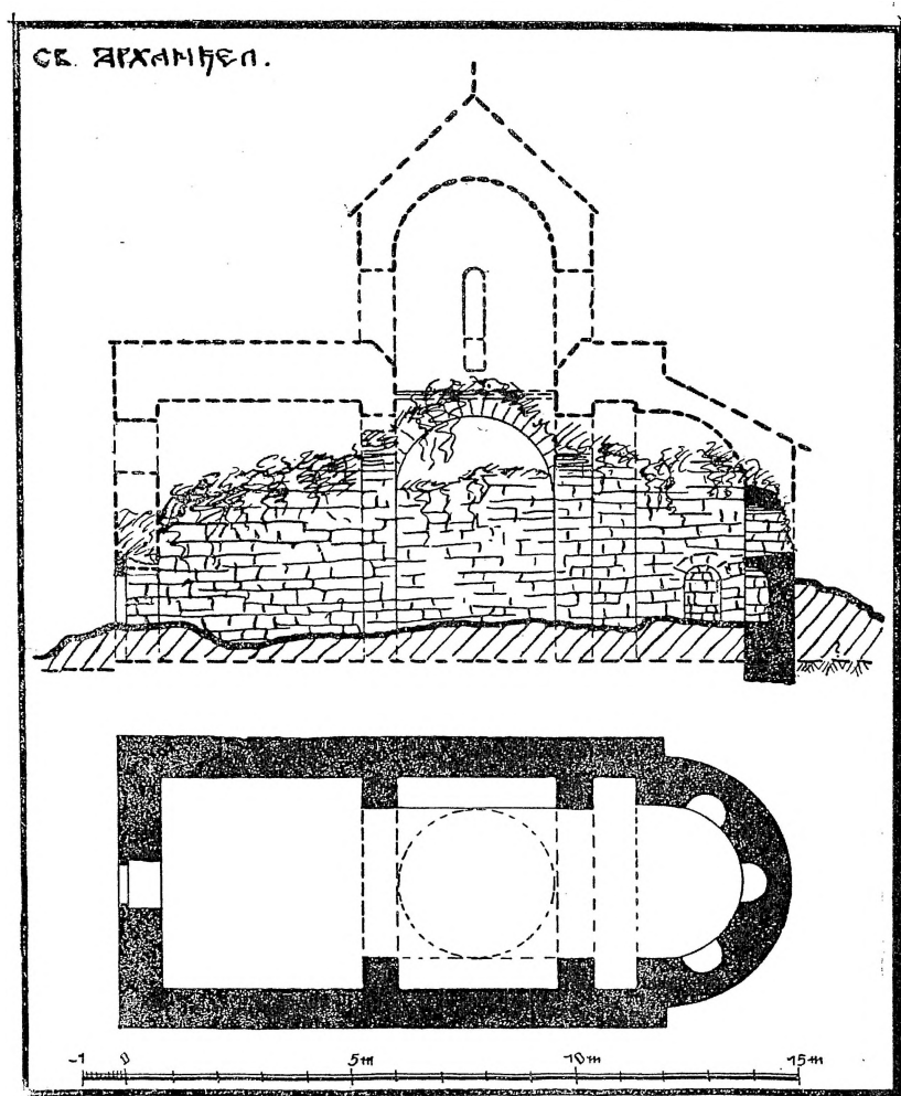
Сл. 8. — Основа и пресек цркве Св. Арханђела на Тари.
