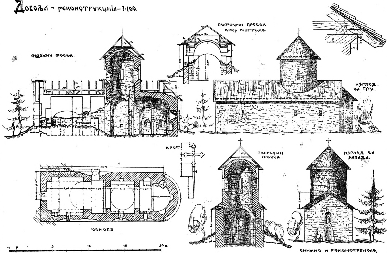
Сл. 4. — Основа, пресеци и реконструкција манастира Довоље.
